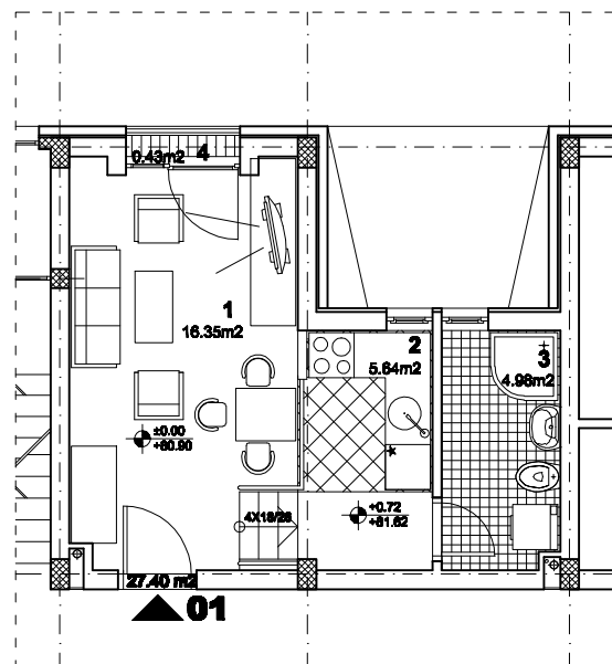
osnova stana R 1:100
