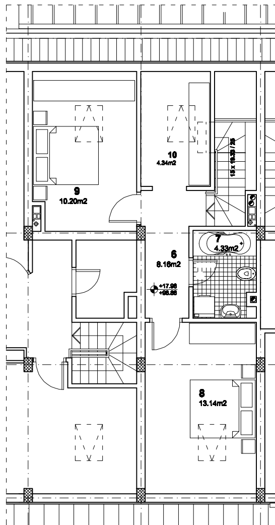
osnova galerije R 1:100
