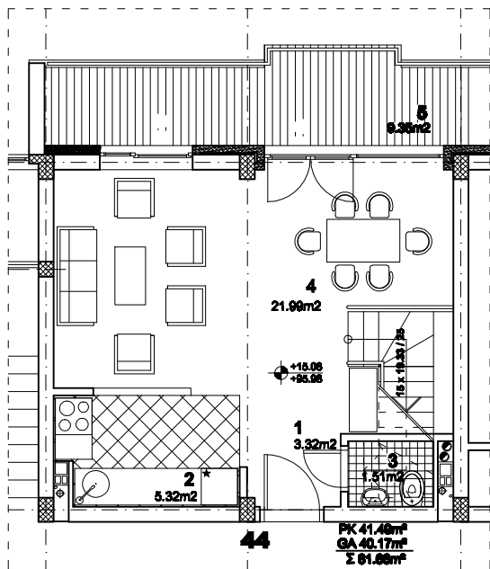
osnova potkrovlja R 1:100
