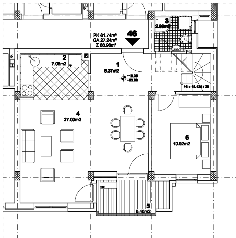
osnova potkrovlja R 1:100
