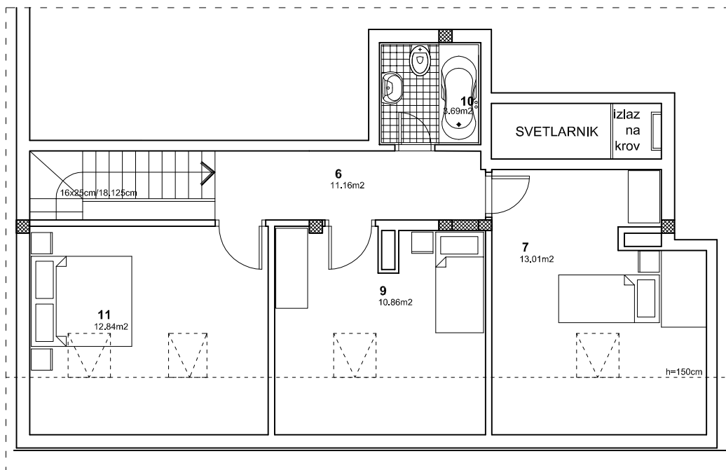
osnova stana R 1:100
