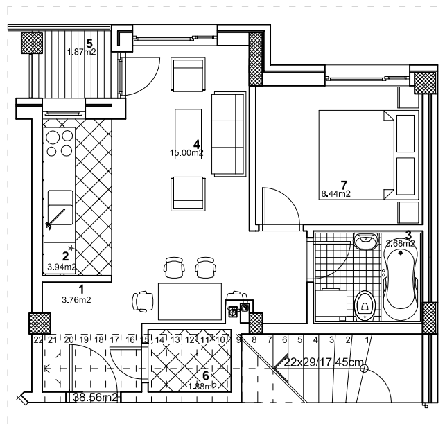
osnova stana R 1:100
