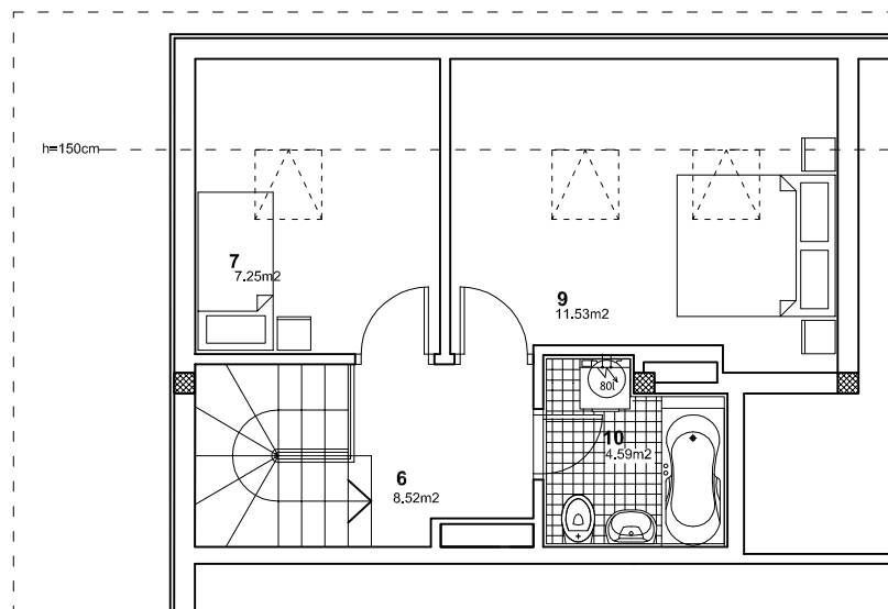
osnova stana R 1:100
