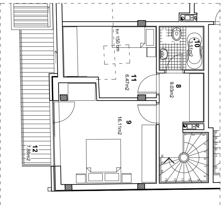
osnova stana R 1:100
