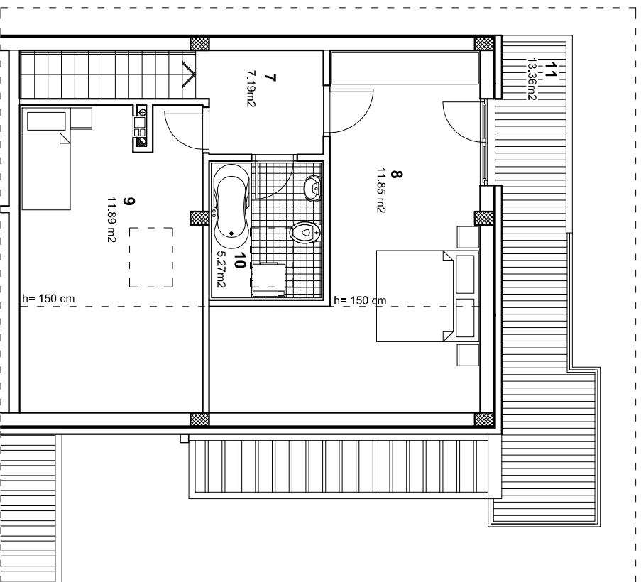
osnova stana R 1:100
