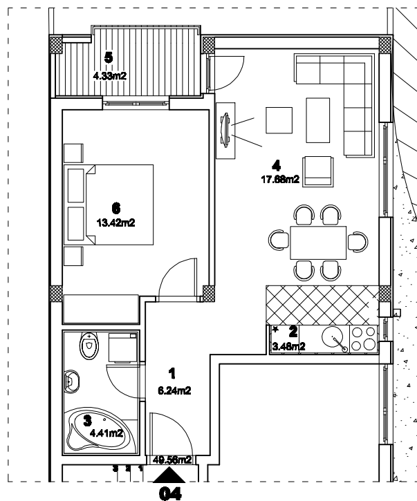
osnova stana R 1:100
