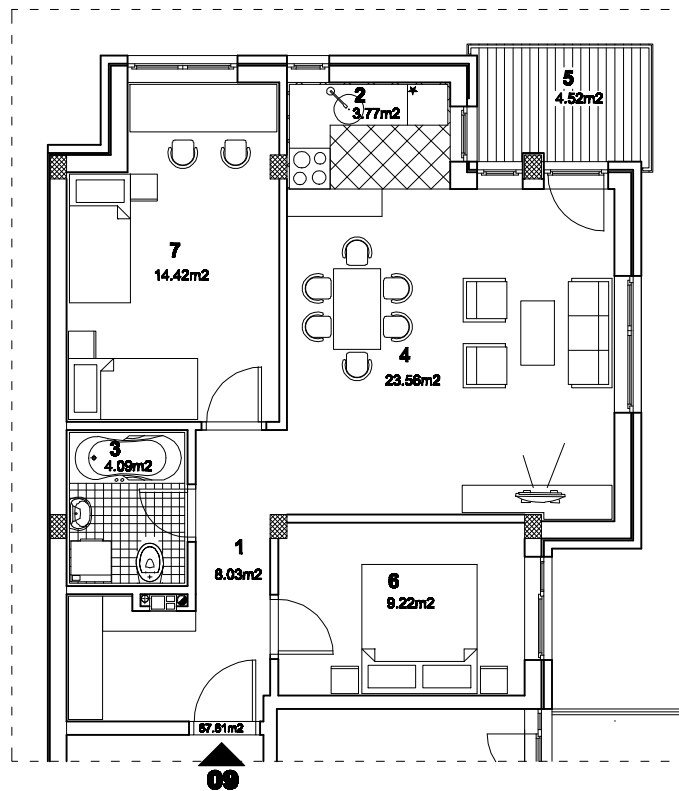
osnova stana R 1:100
